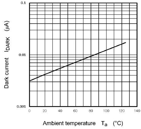
Fig. 11.10 I_{\text{DARK}} - T_a
